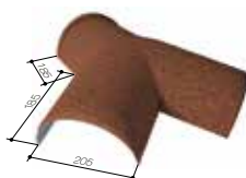
VALBOVÝ ROH „Y“ 205 15-30°
