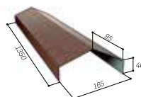
HREBENÁČ DLHÝ CORONA AR95
