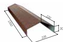
HREBENÁČ DLHÝ CORONA AR130
